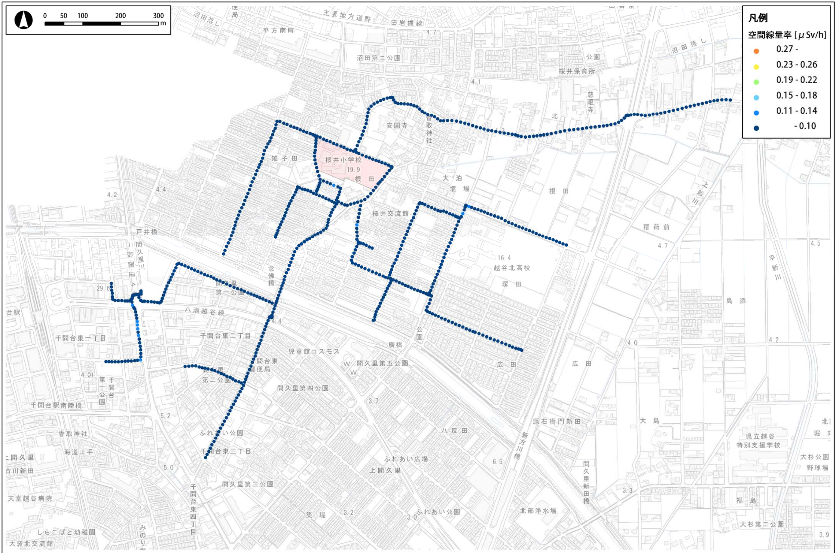
図1 桜井小学校通学路（登校側）における空間線量分布図
