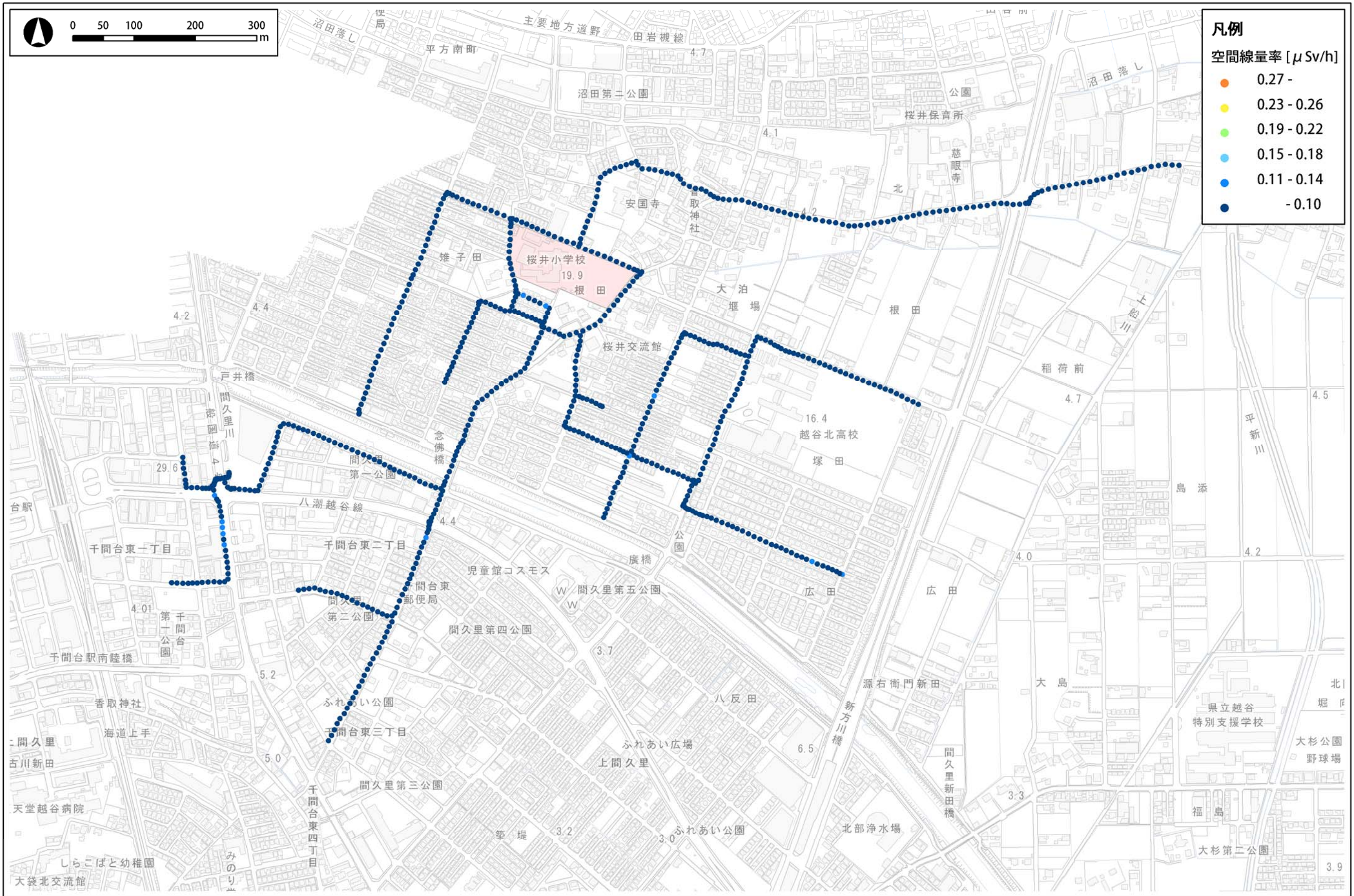
図2 桜井小学校通学路（下校側）における空間線量分布図
