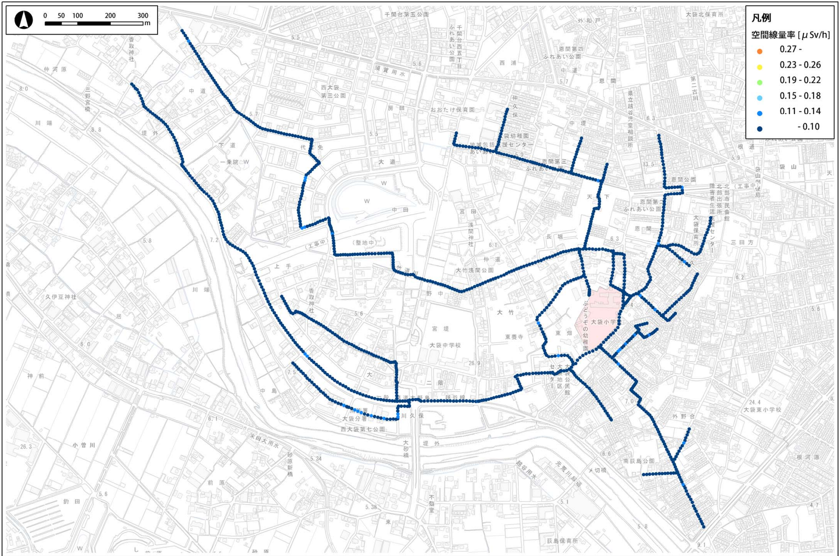
図2 大袋小学校通学路（下校側）における空間線量分布図
