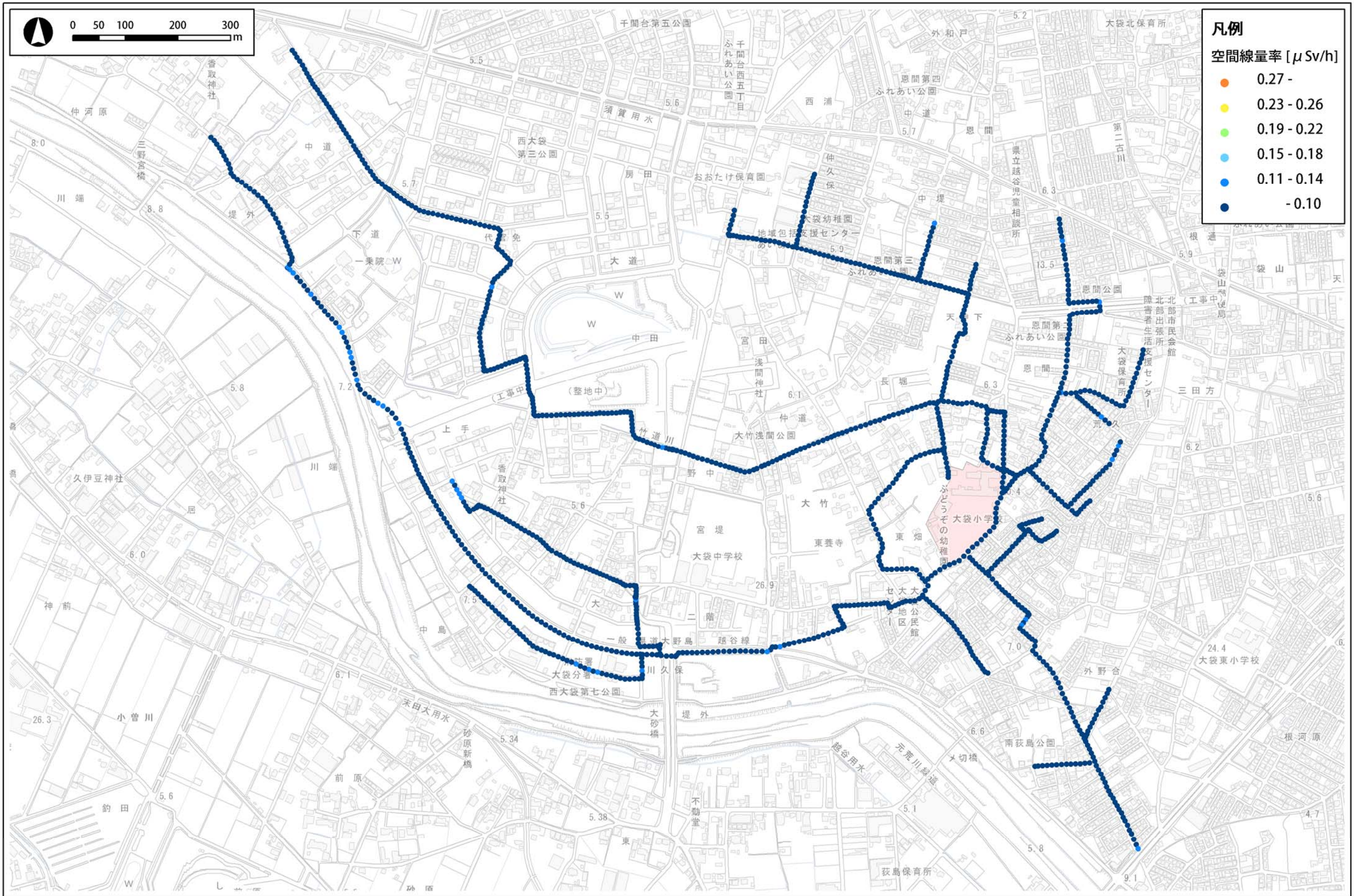
図1 大袋小学校通学路（登校側）における空間線量分布図
