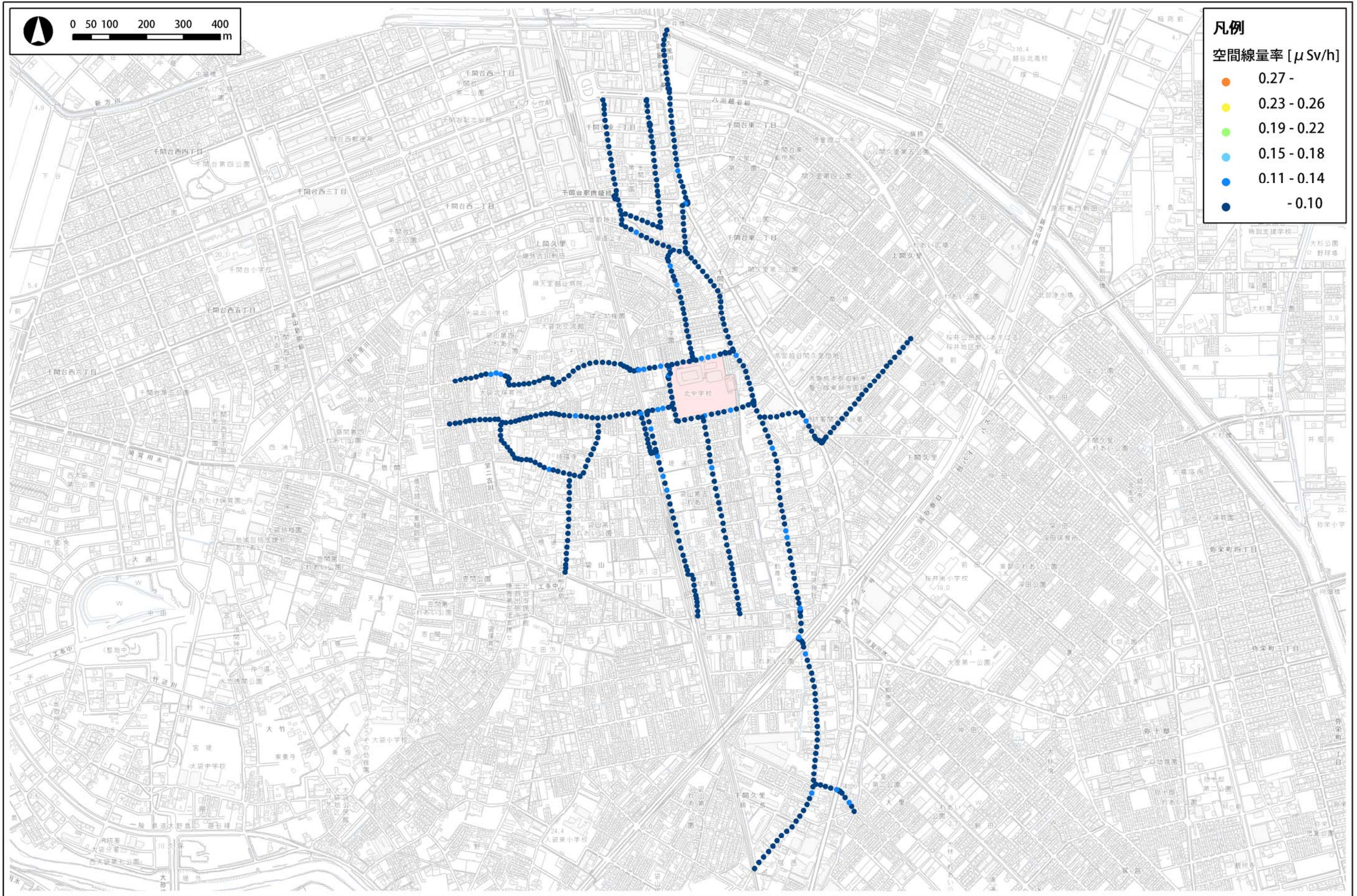
図2 北中学校通学路（下校側）における空間線量分布図
