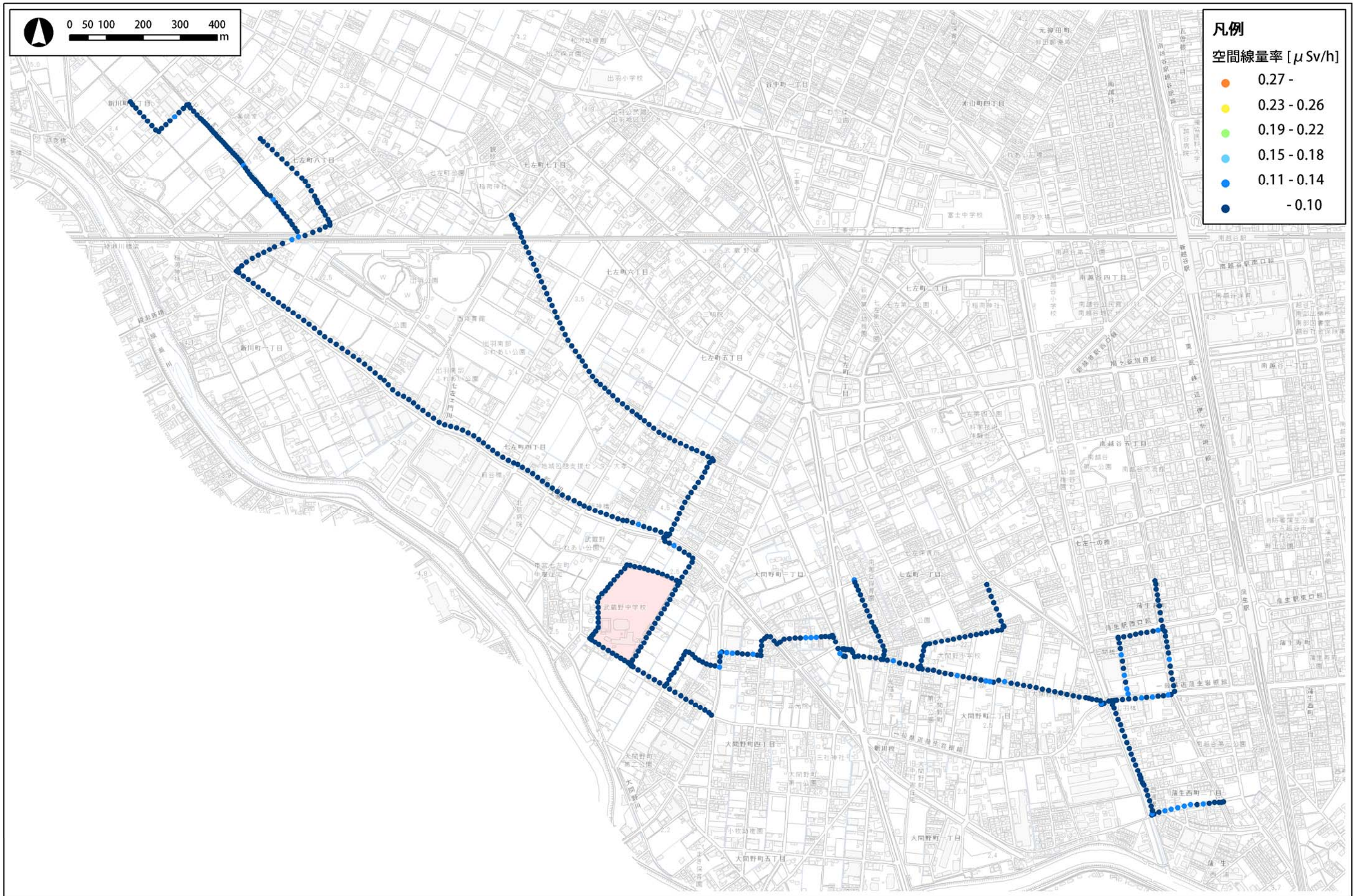
図2 武蔵野中学校通学路（下校側）における空間線量分布図
