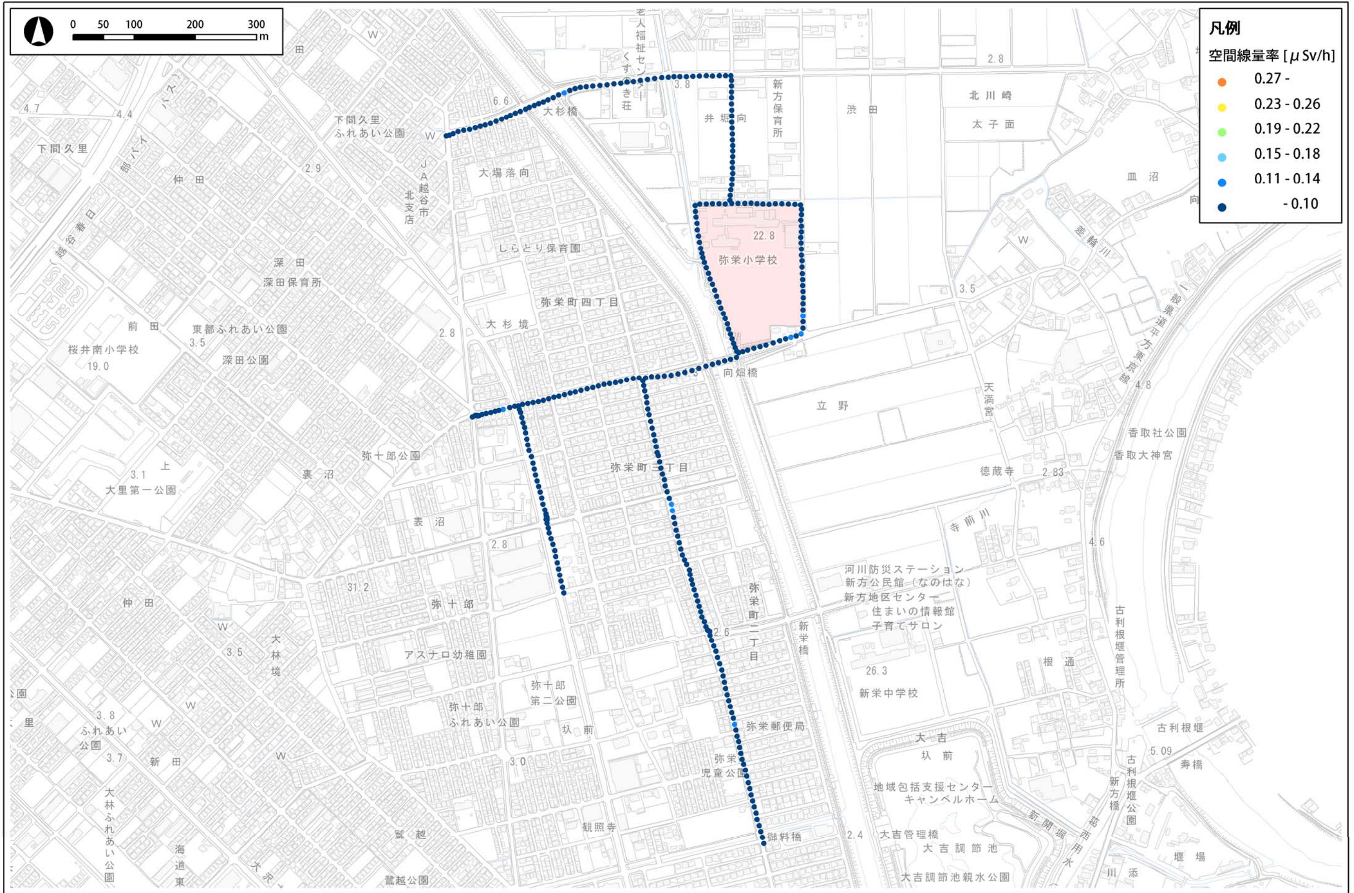
図1 弥栄小学校通学路（登校側）における空間線量分布図
