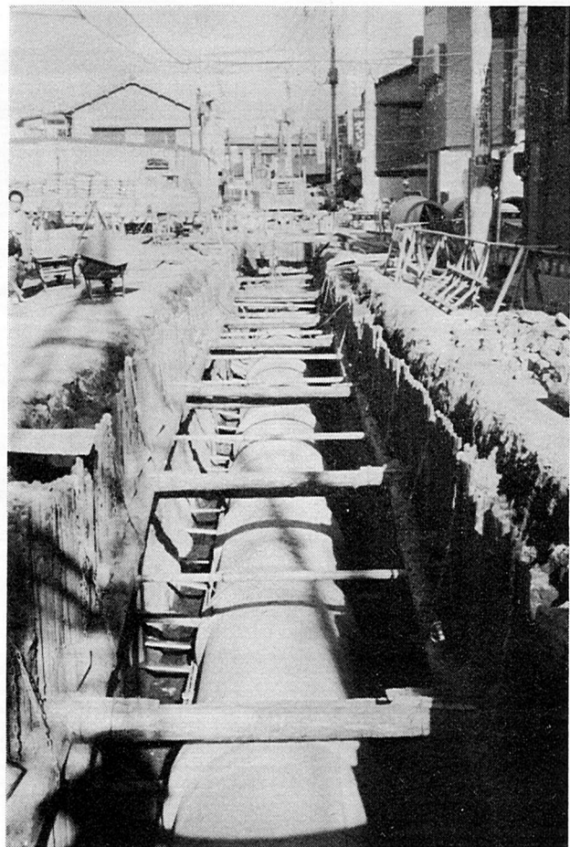
弥生町に埋設された下水管
