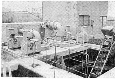
南越谷の仮設ポンプ場
