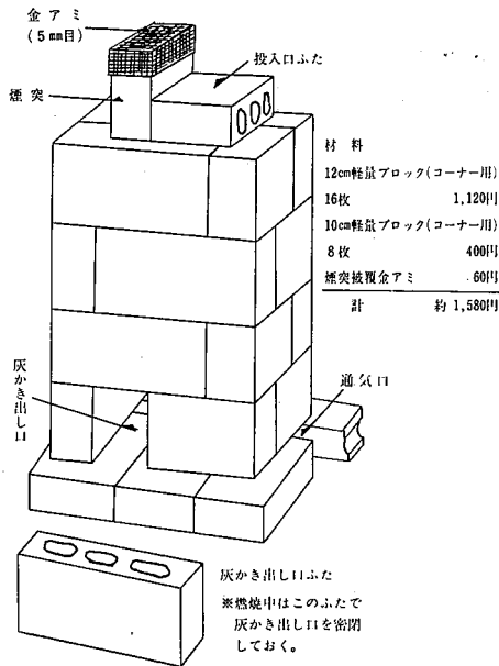
簡易焼却炉完成図
