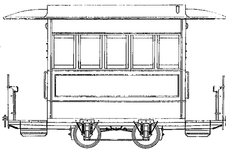
株式千住馬車鉄道會社車臺圖
