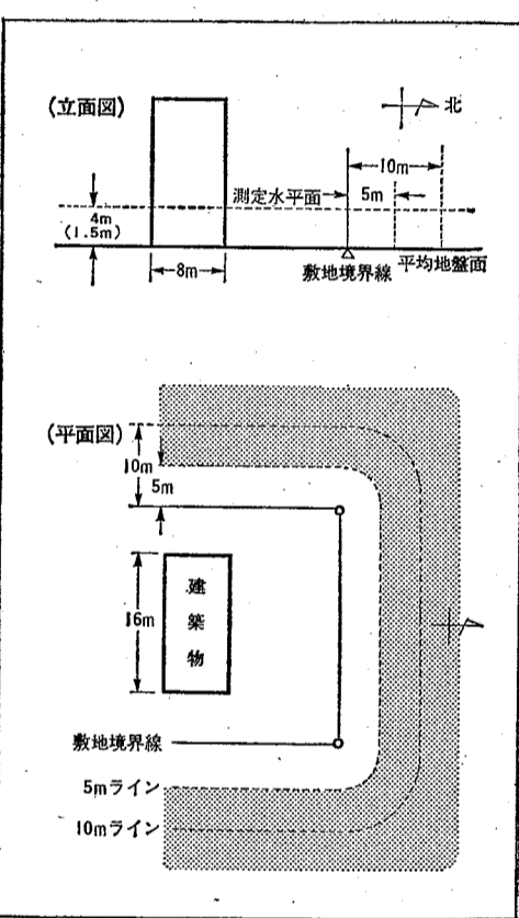
図1 日影を規制する範囲及び測定水平面
