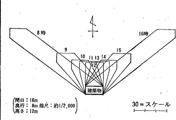
図2 日影図
