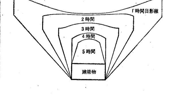
図3 日影時間図
