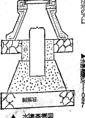
▲水準器の構造
