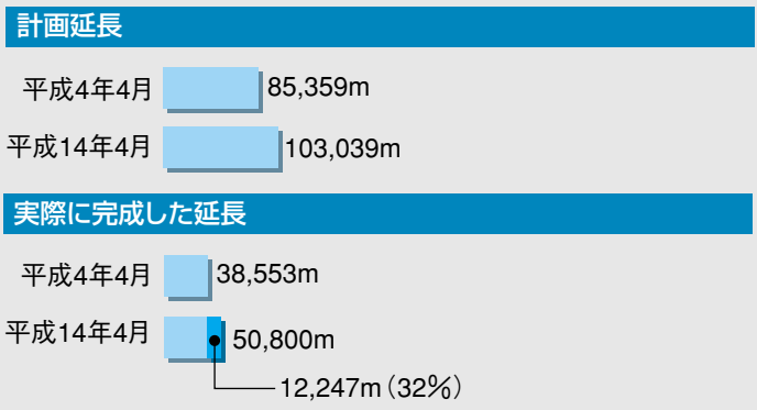
（表5） 都市計画街路整備の推移
