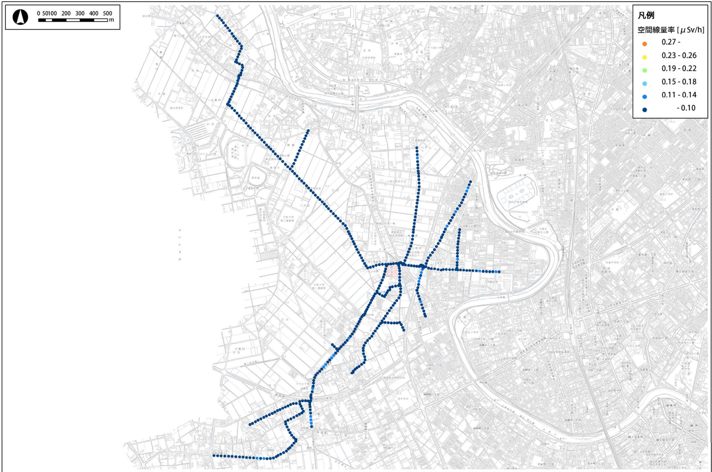
図1 荻島小学校通学路（登校側）における空間線量分布図
