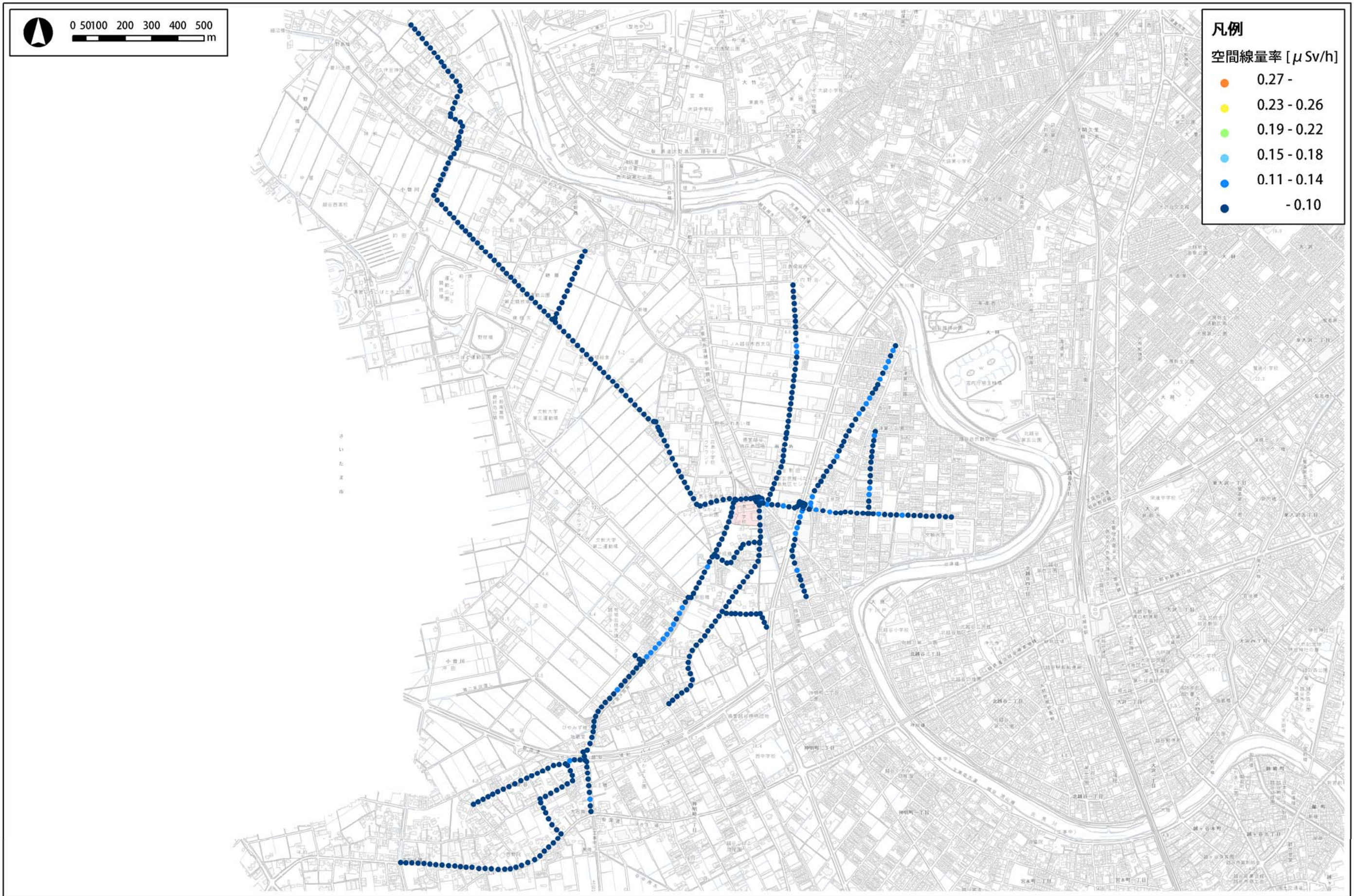
図2 荻島小学校通学路（下校側）における空間線量分布図
