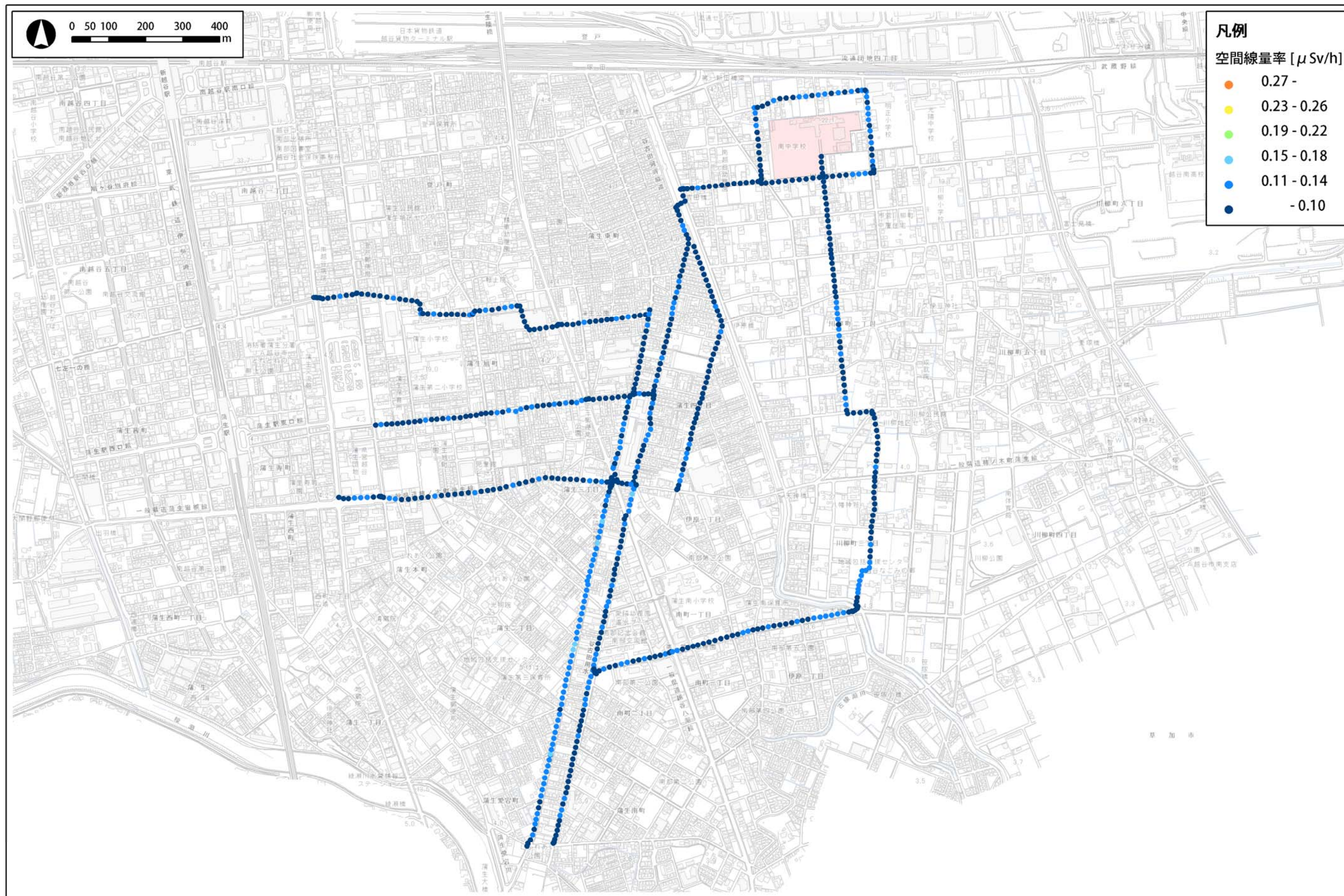
図2 南中学校通学路（下校側）における空間線量分布図
