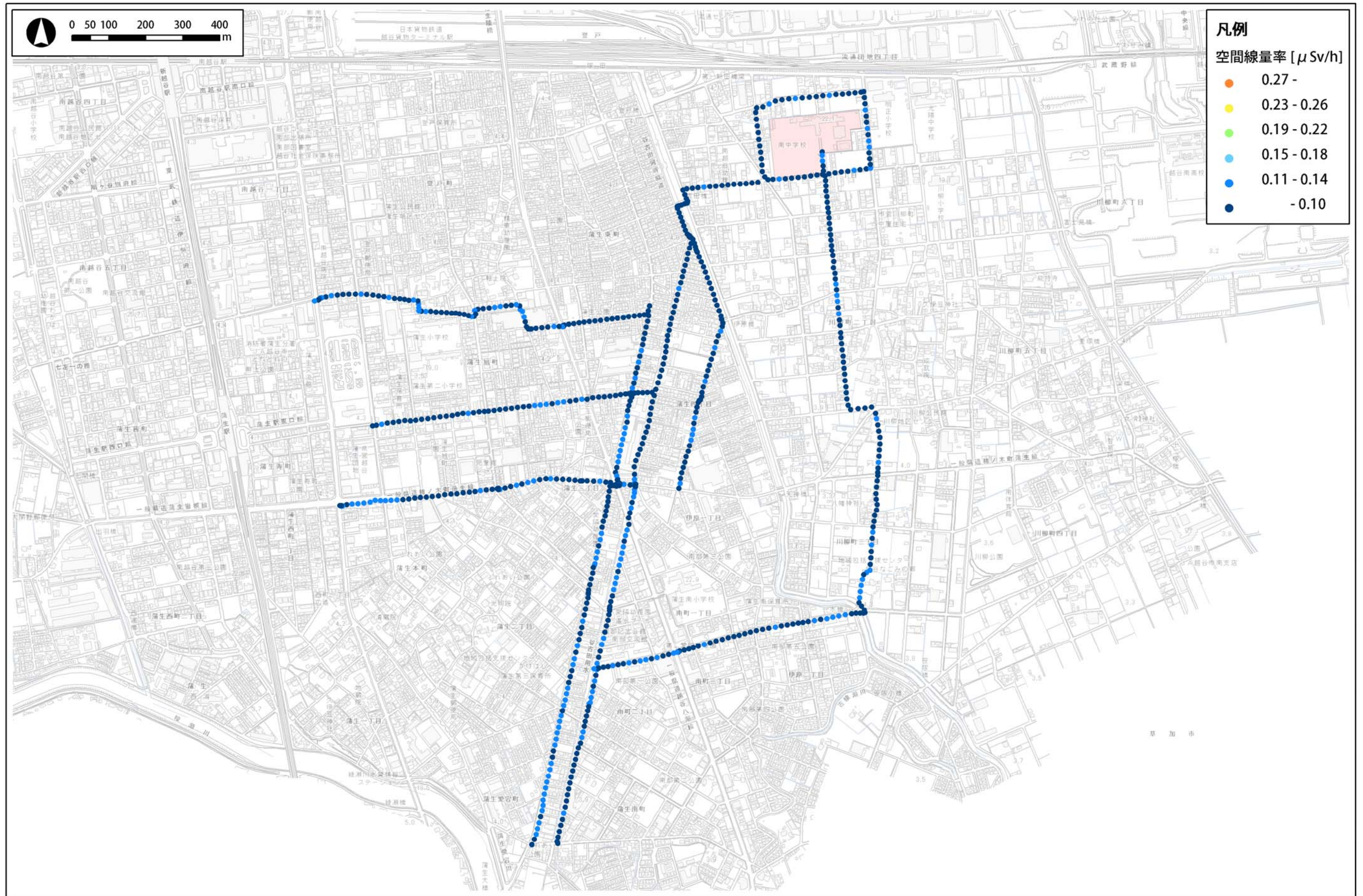
図1 南中学校通学路（登校側）における空間線量分布図
