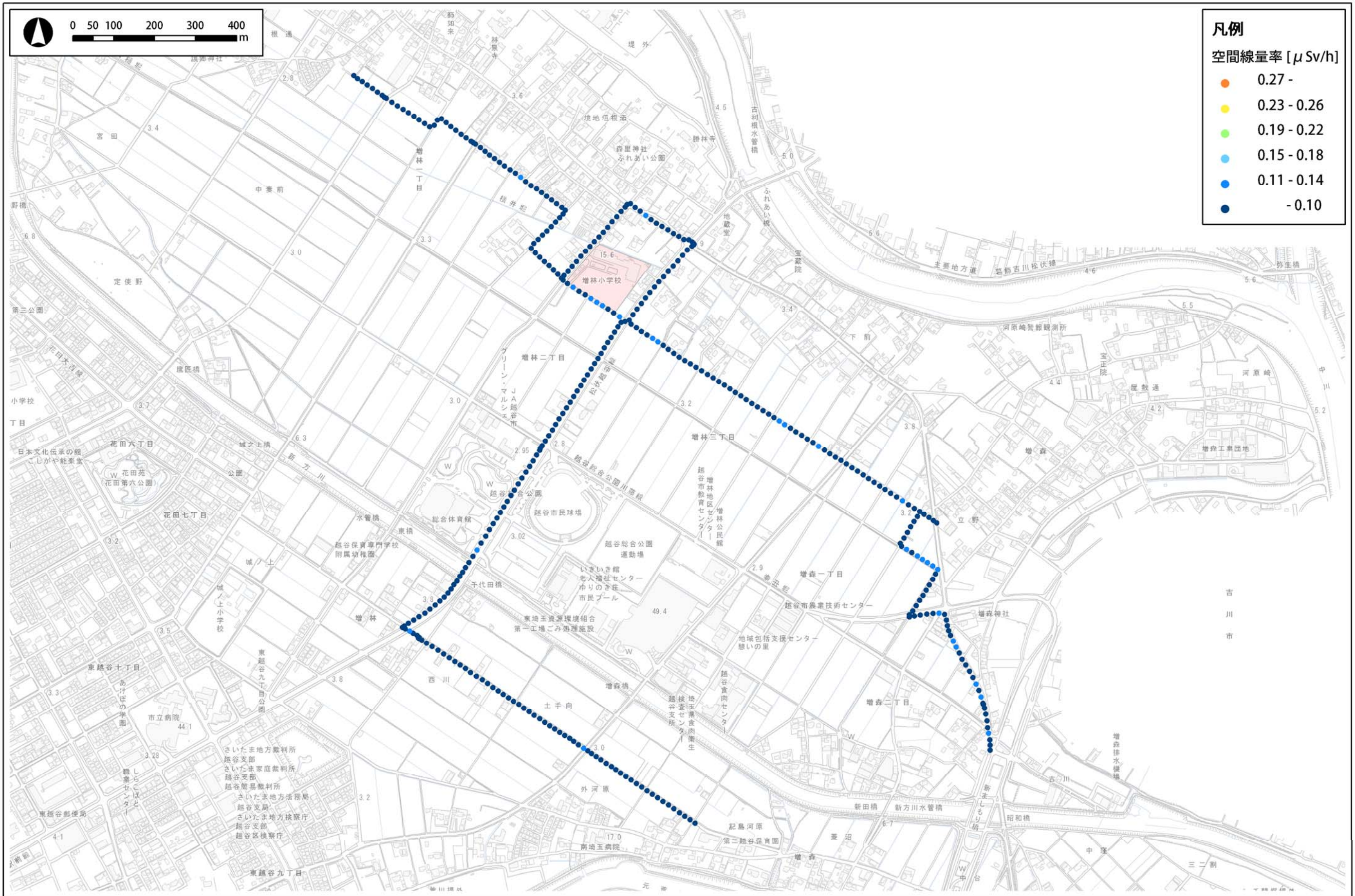
図2 増林小学校通学路（下校側）における空間線量分布図
