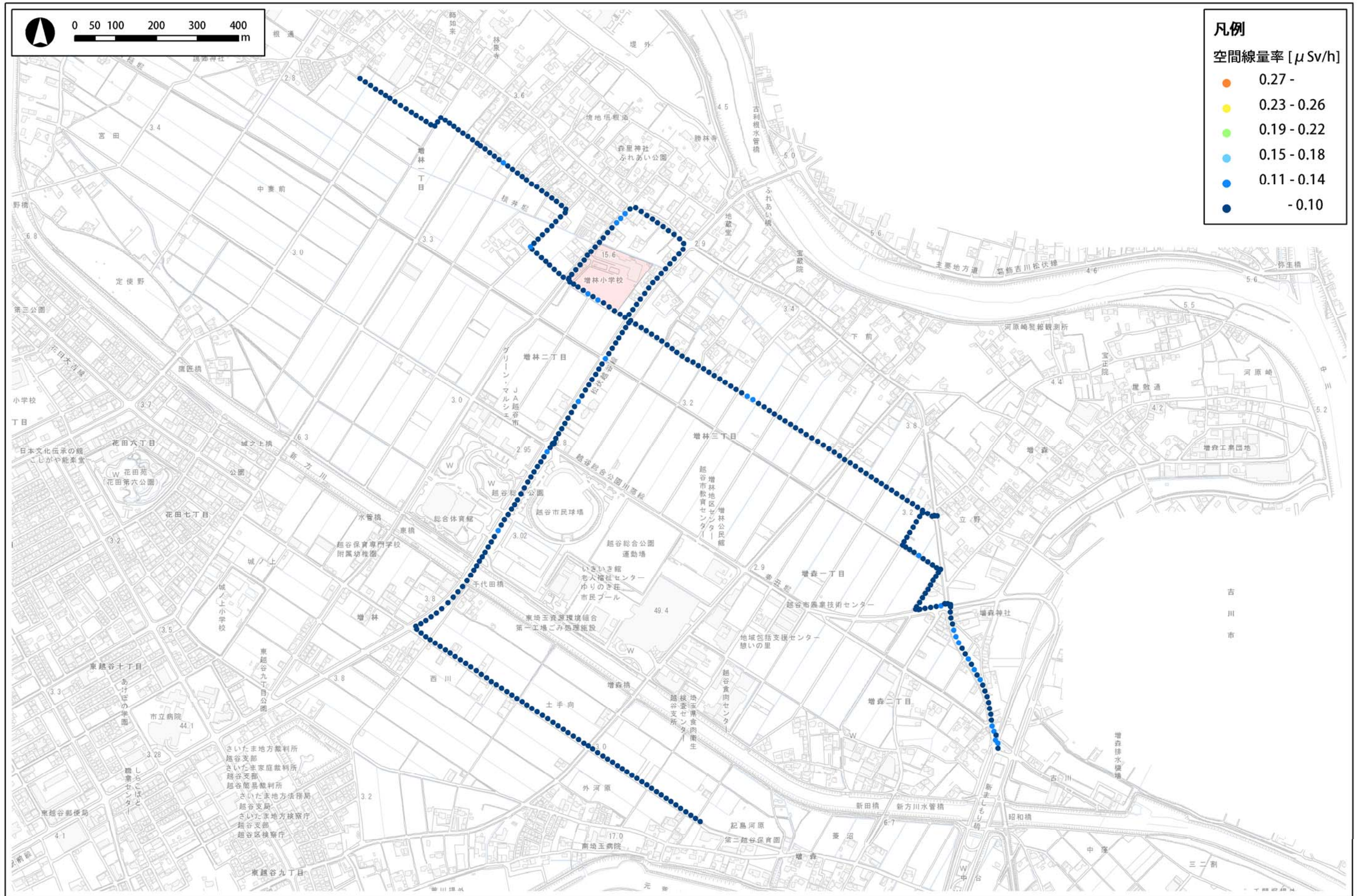
図1 増林小学校通学路（登校側）における空間線量分布図
