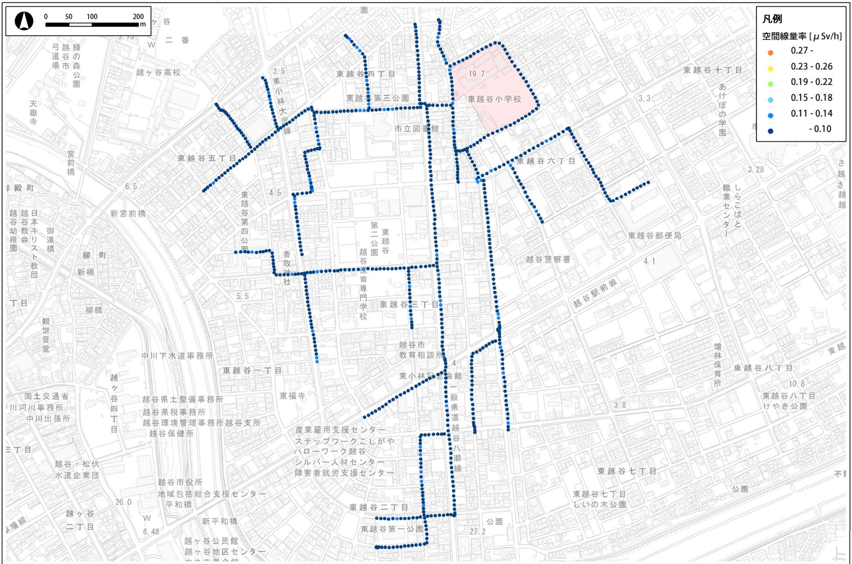
図1 東越谷小学校通学路（登校側）における空間線量分布図
