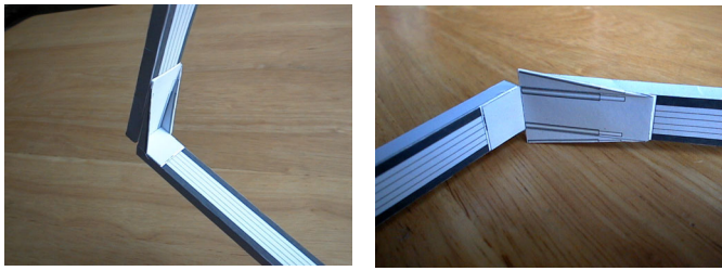
ストッパー完成写真
