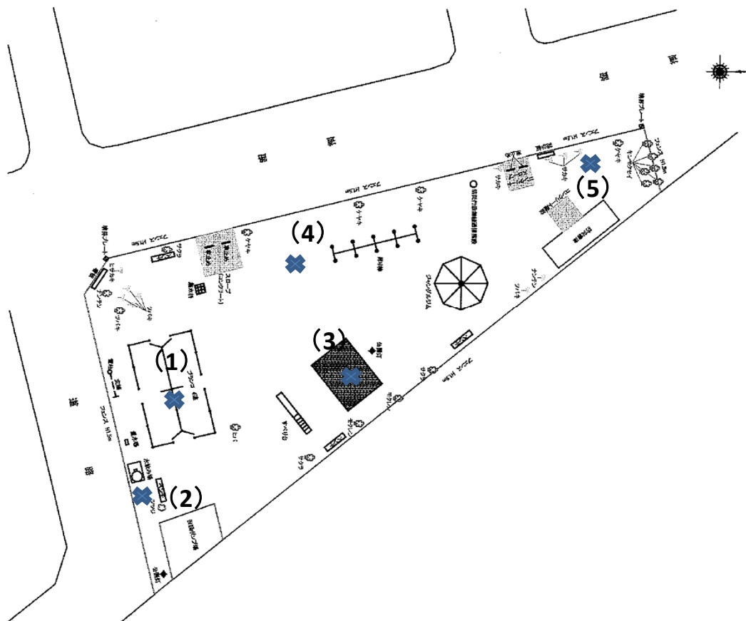
平面図 B-1
