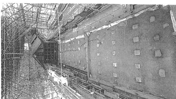
骨組みの解体を終えた田子櫓・七間櫓（南から）
