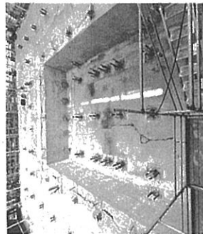
土間部コンクリート基礎の撤去前
