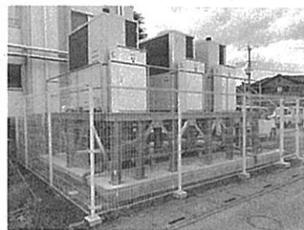
浸水に備えたエアコン室外機の設置
