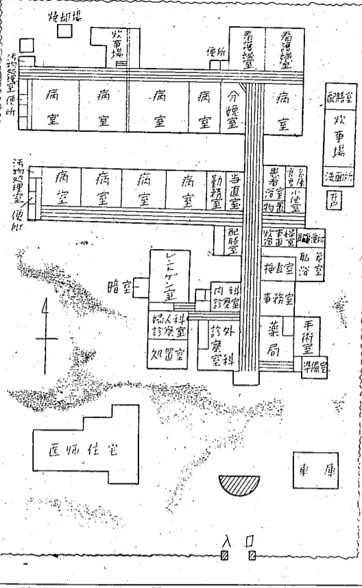
越谷町東武病院平面図
