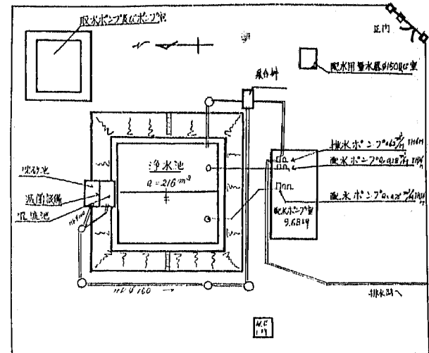
浄水場平面図
