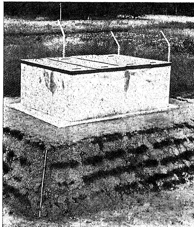
水源用深井戸—深さ260メートル，水中モーターで汲み上げる
