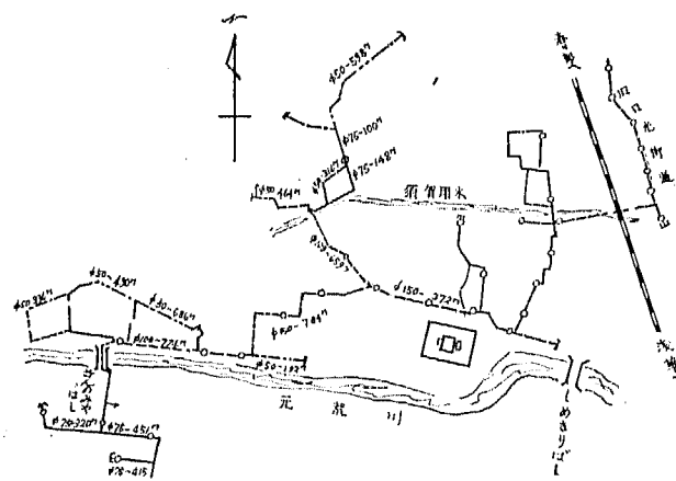
配水管布設見取図
