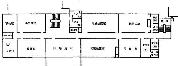
(二階平面図)
