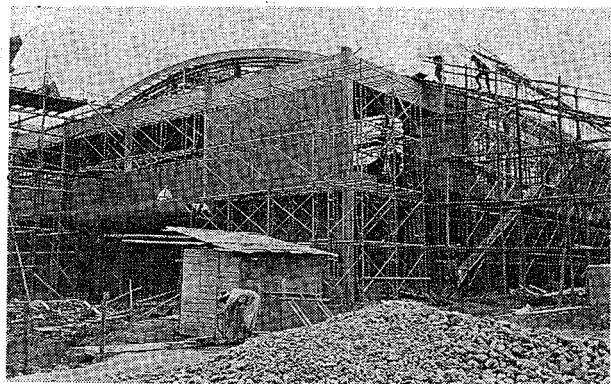
いま増築中の体育館は、鉄骨造り2階建て延べ床面積は1,200平方メートル。2階に観覧席。工事費は4,195万円、今月末にできあがります。
