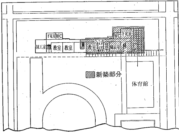
蒲生小文教場新築見取図
