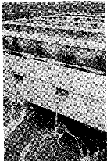
2次曝気槽活性汚泥の処理、消毒が行なわれる
