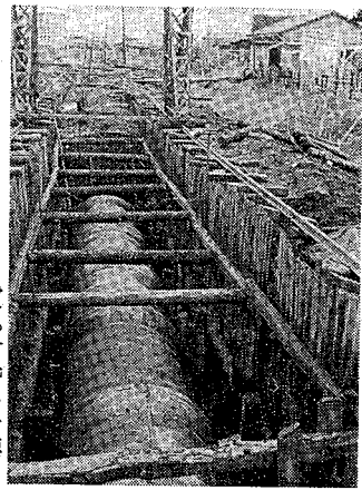
下水道管の敷設工事
