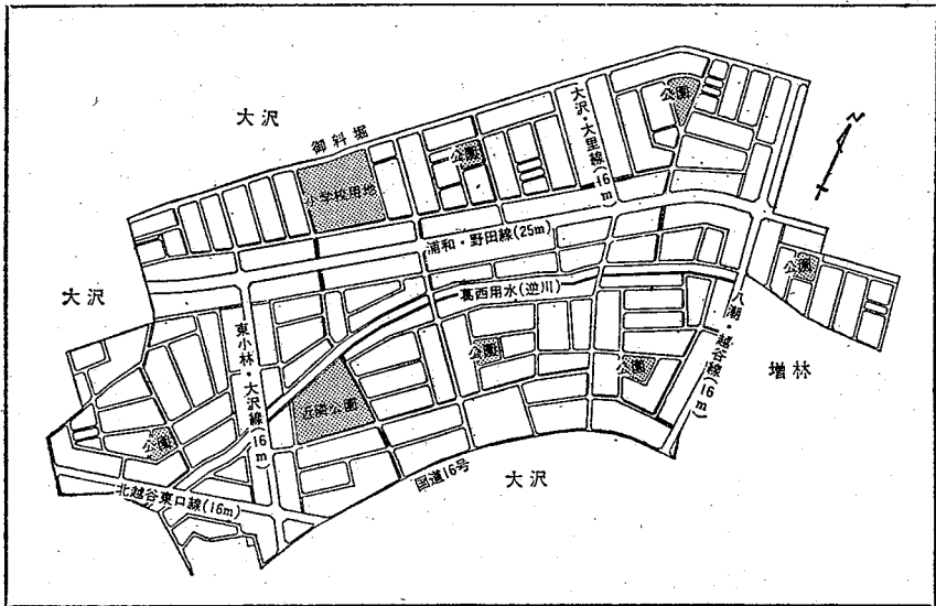
鷺高土地区画整理事業街路計画図
