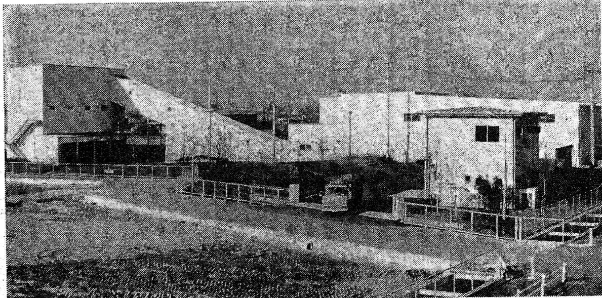
一日約二十三トンの粗大ゴミを選別処理 この粗大ゴミを選別処理センターで、破砕機を出ると粉々に処理する粗大ゴミ処理センター
