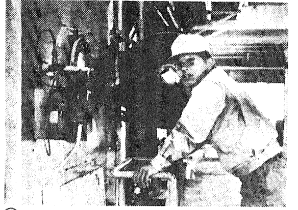
④ ピットからゴミはクレーンで取り入れます。ここで分別から出る生ゴミなど燃えるゴミが燃やされます。ゴミを燃やすための燃料に補助用に使われています。特に夏のゴミは水分が多いので、重油の使用量も増えるということです。
