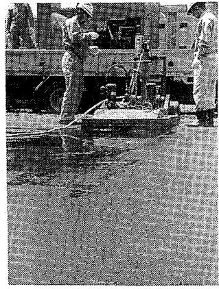
ガラスなどの細粒を舗装の骨材に利用
