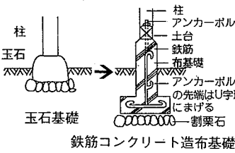
鉄筋コンクリート造布基礎
