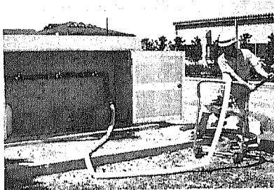
耐震型緊急用(飲料用)貯水槽
