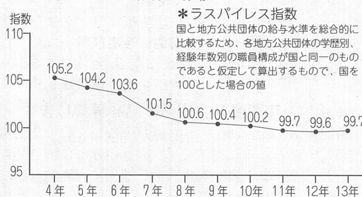
図1 ラスパイレス指数の推移
