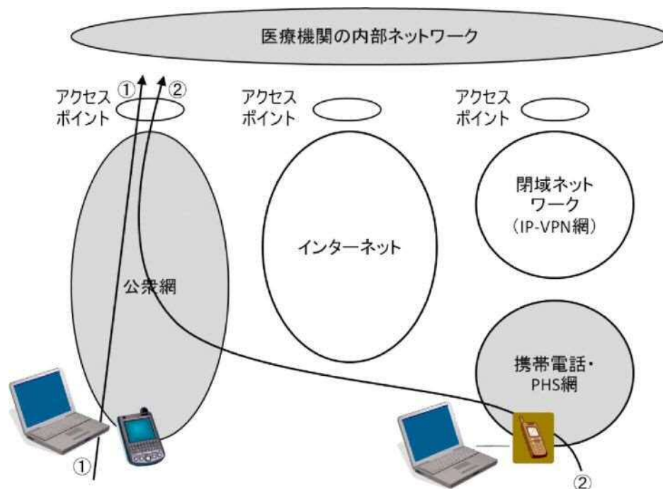
図 B-2-㉞ モバイル環境における接続形態（公衆網経由）
