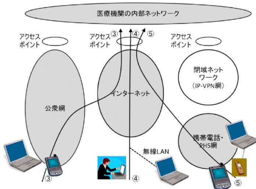
図 B-2-⑥ モバイル環境における接続形態（インターネット経由）
