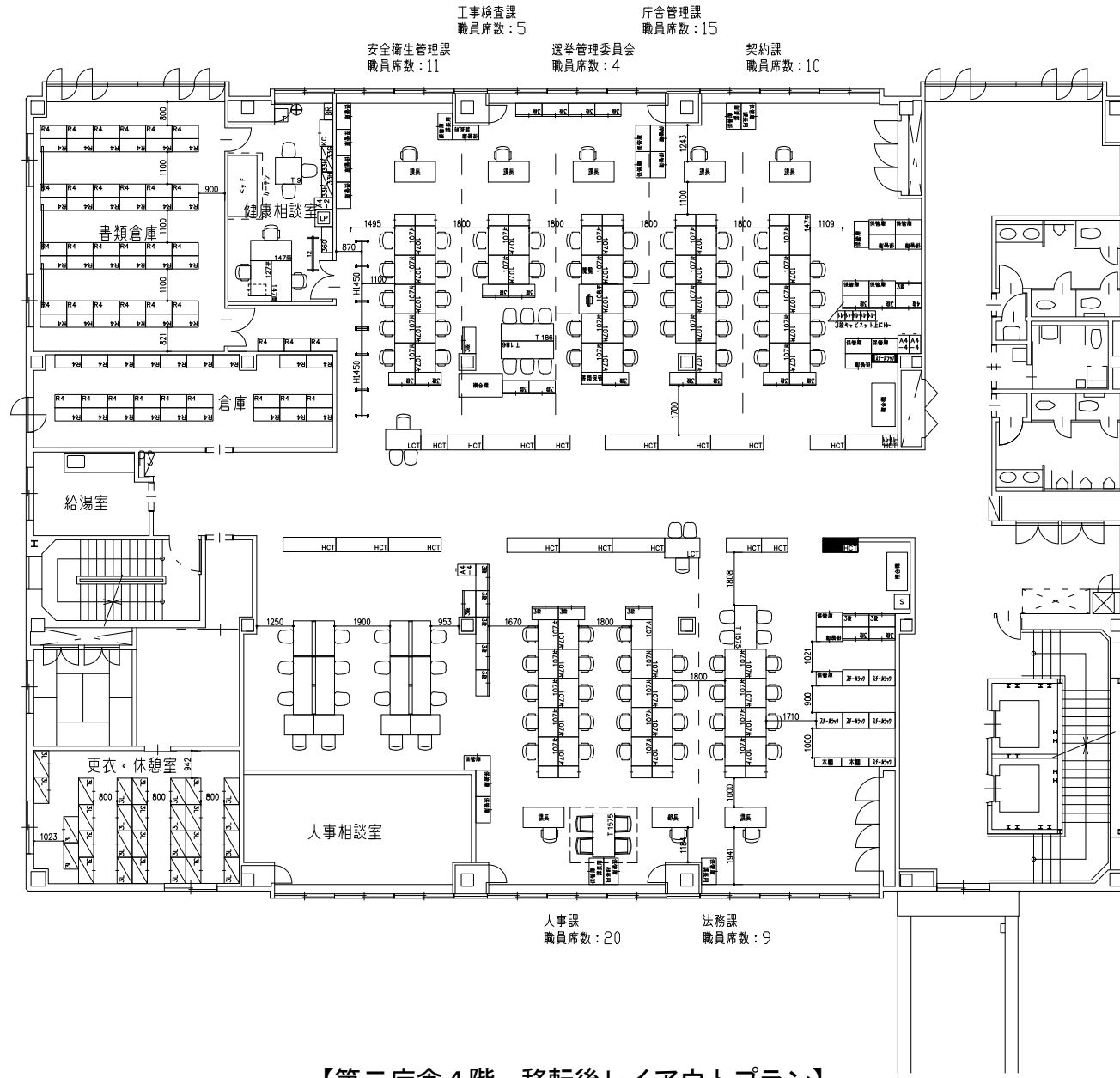
【第二庁舎4階 移転後レイアウトプラン】
