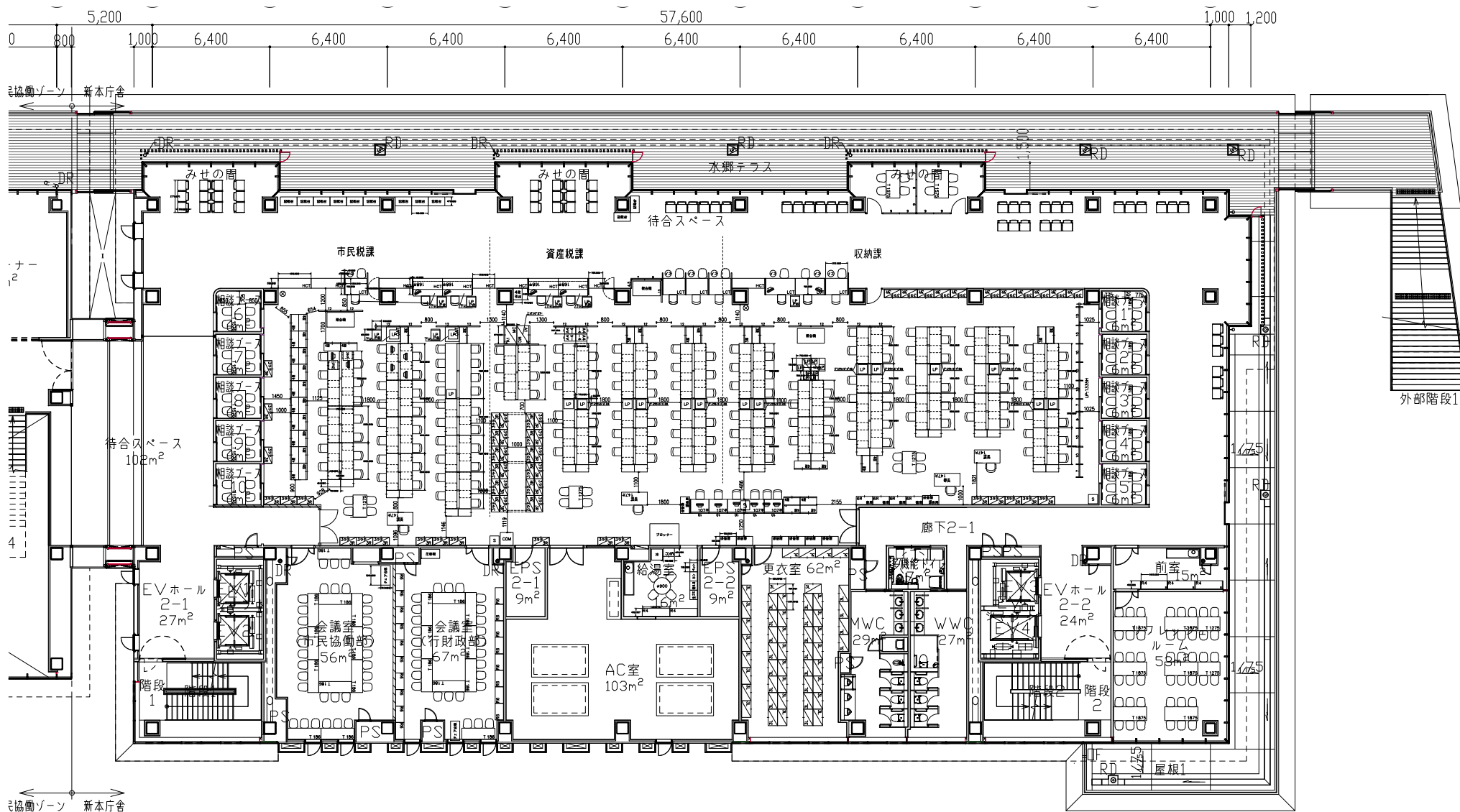
【新本庁舎2階 移転後レイアウトプラン】
