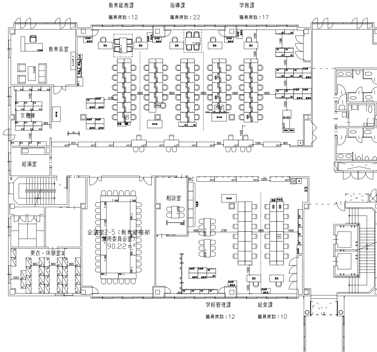
【第二庁舎3階 移転後レイアウトプラン】
