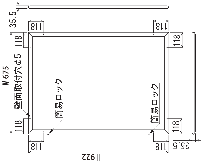
意匠図
