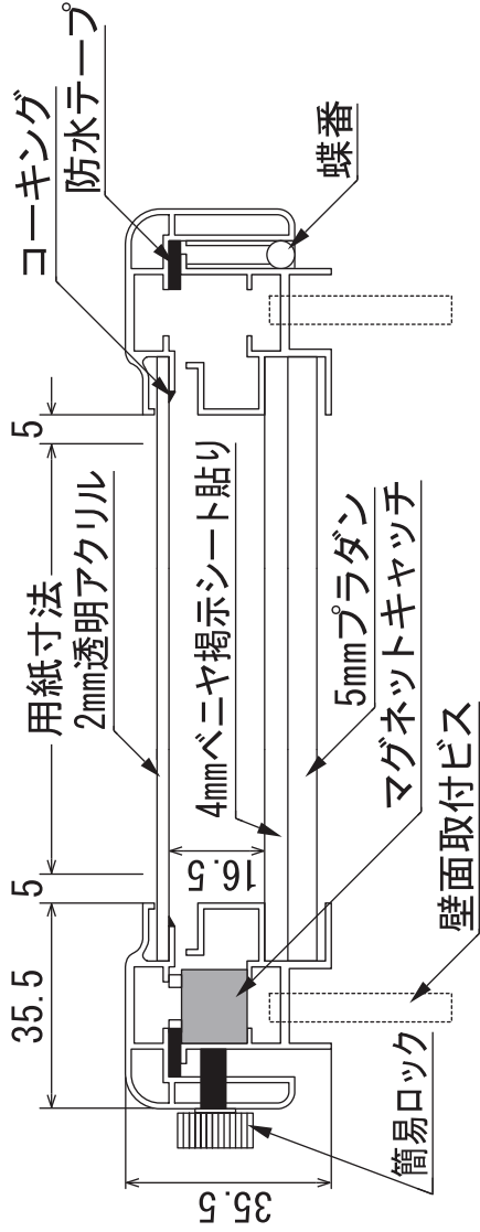
断面図
