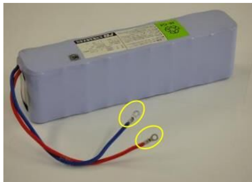
電極端子部露出の例 (出典:JBRC)
