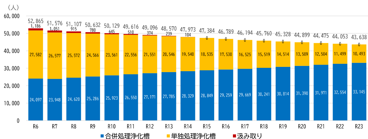
図4-3 浄化槽処理区域の将来推計結果（直近5年間実績に基づく）
