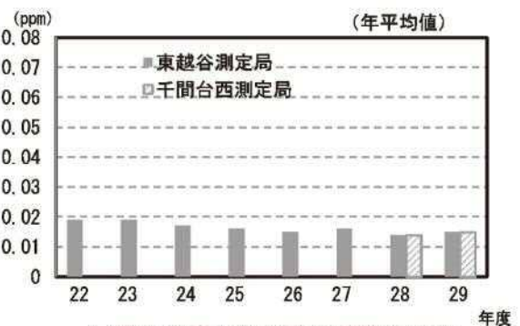
二酸化窒素の年平均値の経年変化
