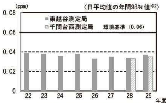
二酸化窒素の日平均値の経年変化
