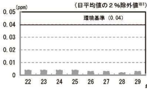
二酸化硫黄の日平均値の経年変化
