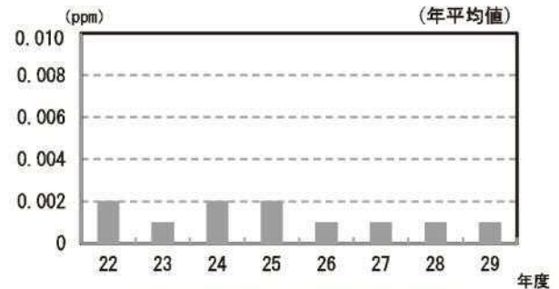
二酸化硫黄の年平均値の経年変化
