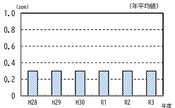
一酸化炭素の年平均値の経年変化
