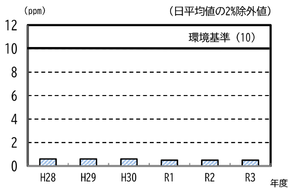
一酸化炭素の日平均値の経年変化
