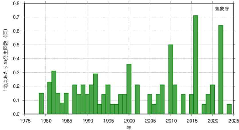
図 埼玉県内アメダス（15か所）における時間雨量 50mm 以上降雨回数 出典)「関東甲信地方のこれまでの気候の変化(観測結果)」(東京管区気象台ホームページ)
