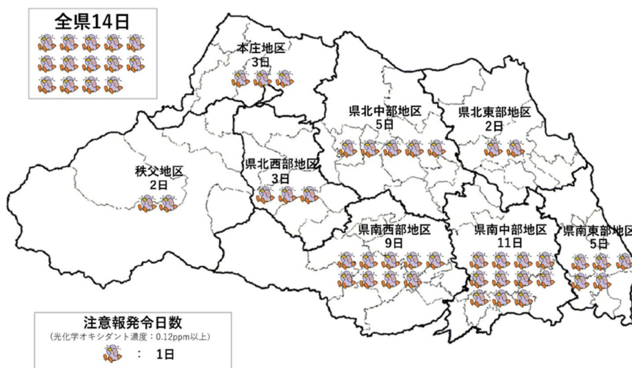
図 地区別光化学スモッグ注意報発令日数 出典) 「令和6年(2024年) 光化学スモッグの発生状況について」(埼玉県)
