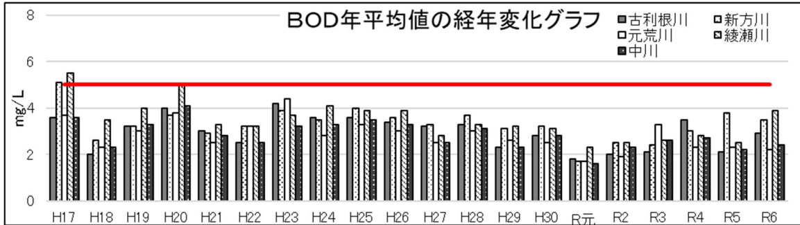
図 本市における河川のBODの経年変化 出典)「令和7年度(2025年度)越谷市環境白書」
