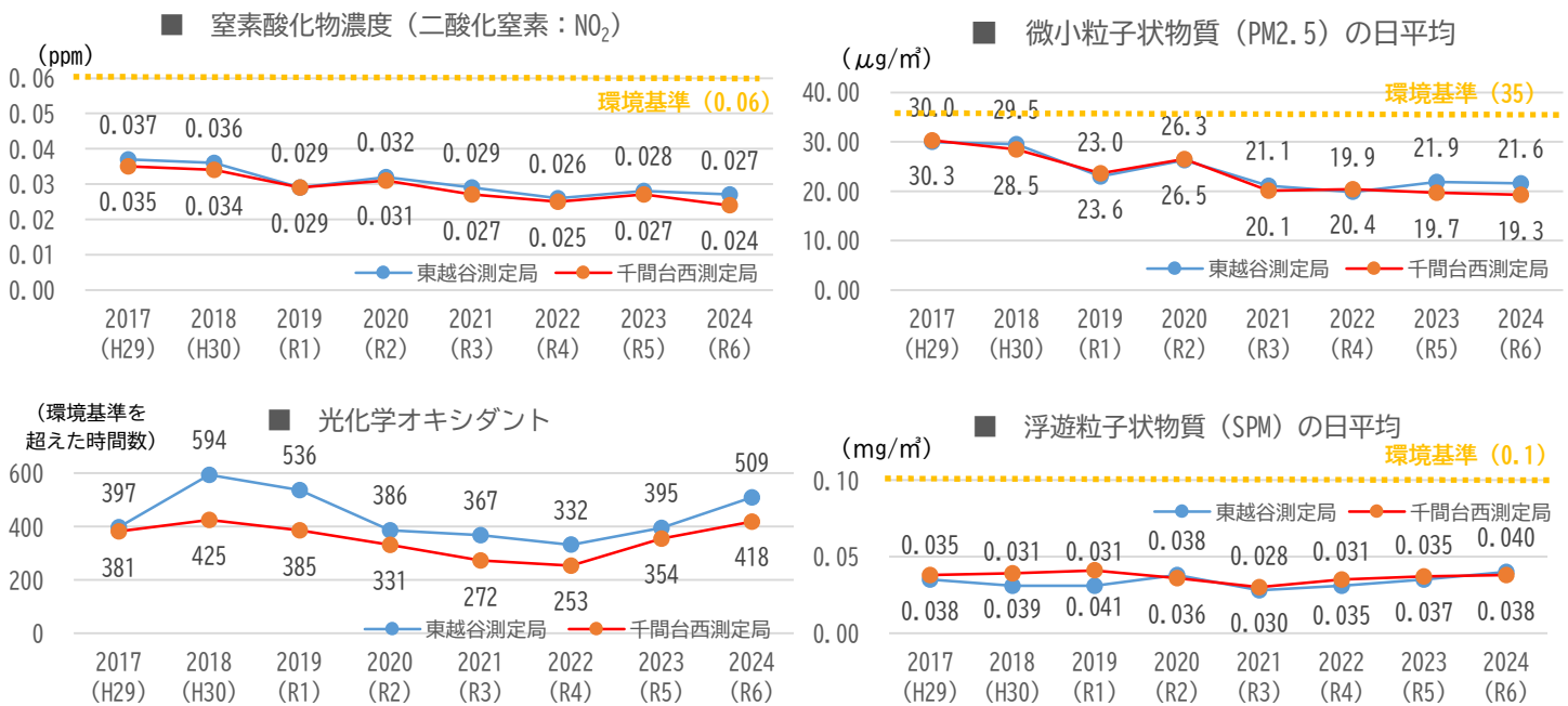
図 本市における大気汚染状況の経年変化 出典) 越谷市
