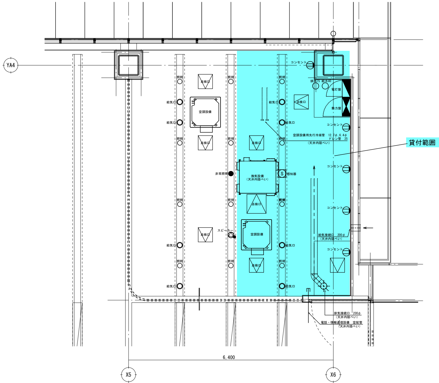
A 工事設備図 (カフェ) S=1/50 (A3)
