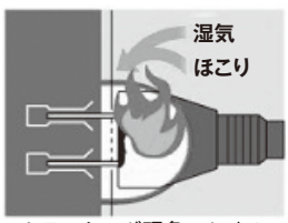
トラッキング現象のしくみ
