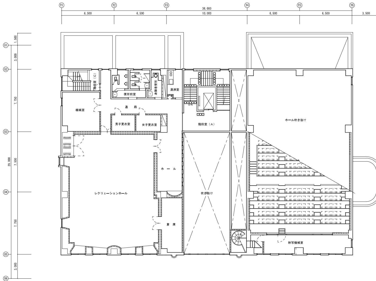
4 階 平 面 図 S = 1 / 1 5 0
