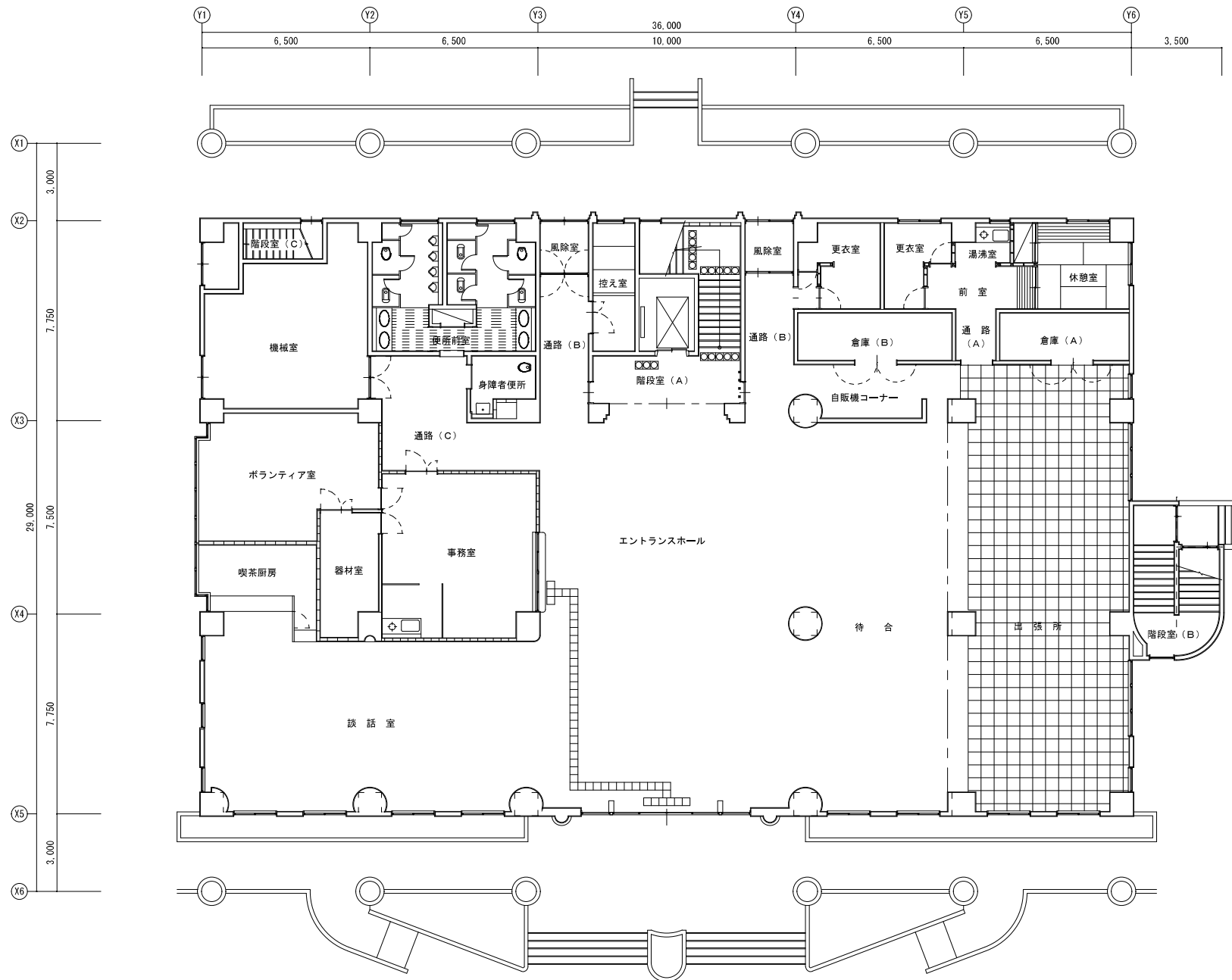
1 階 平 面 図 S = 1 / 1 5 0
