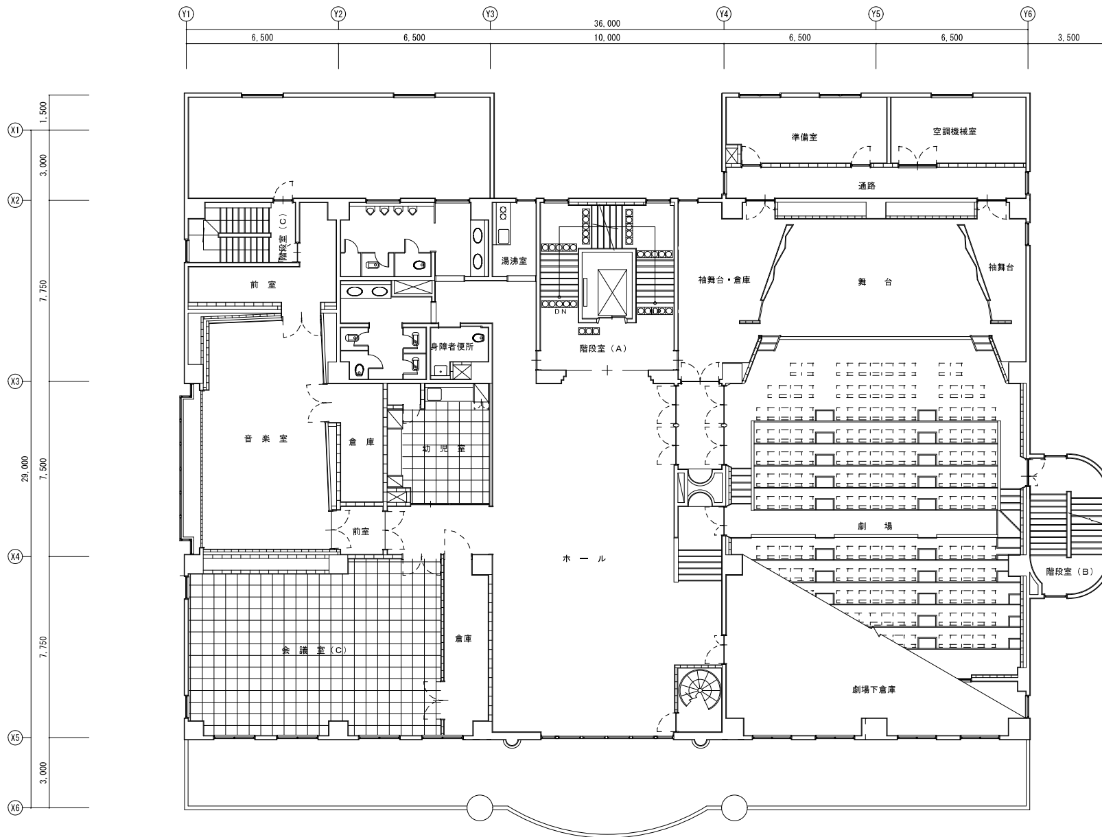
3 階 平 面 図 S = 1 / 1 5 0
